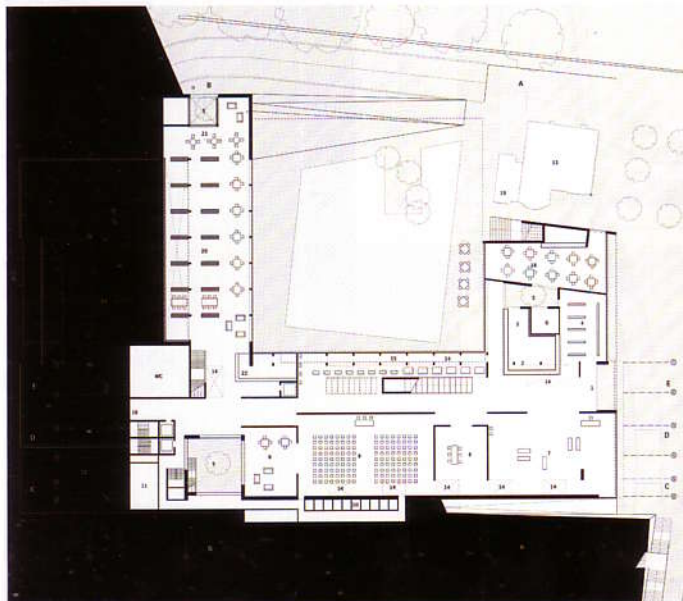
Level 1 M. 1:1.000
